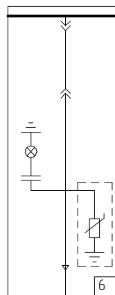
6 Шкаф с разъединителем. Ввод/вывод кабелем вниз.
