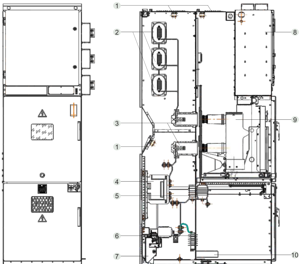
Рис. 4.5 Разрез КРУ
