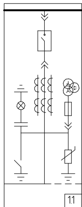
Шкаф с силовым выключателем и измерительным тр-ом. Ввод/вывод шинами сбоку.
