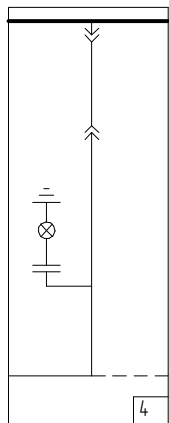
Шкаф секционного разъединителя. Ввод/вывод шинами сбоку.
