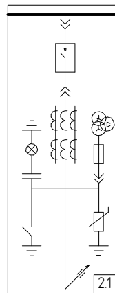
Шкаф с силовым выключателем и измерительным тр-ом. Ввод/вывод шинами сзади.
