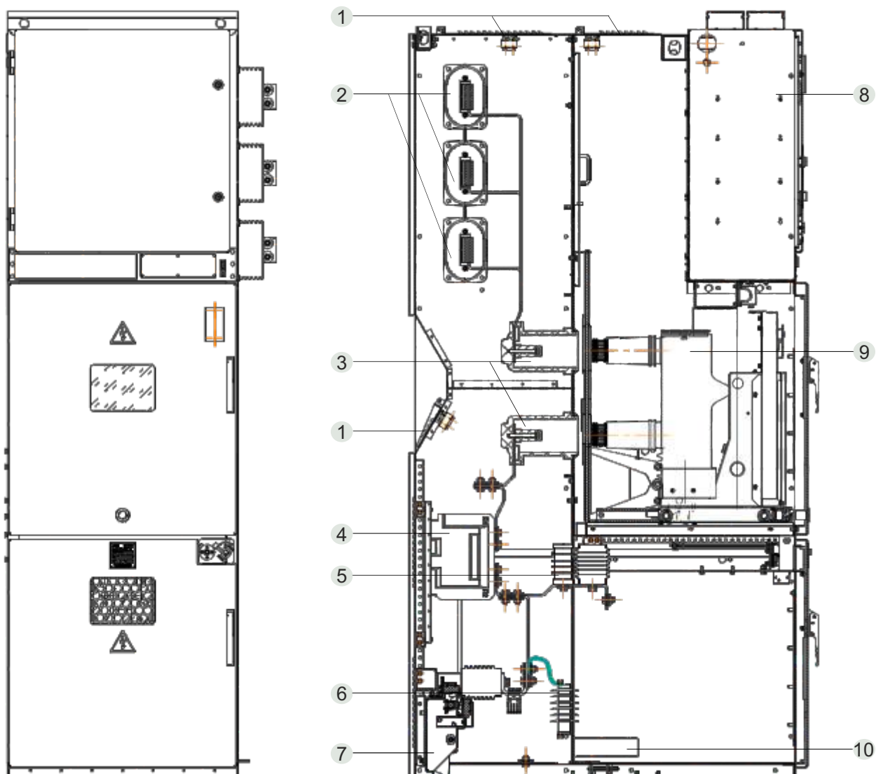
Рис. 4.5 Разрез КРУ
