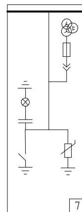
7 Шкаф с шинным заземлителем и измерительным тр-ом.
