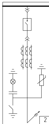
Шкаф с силовым выключателем. Ввод/вывод шинами сзади.
