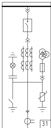
Шкаф с силовым выключателем и измерительным тр-ом. Ввод/вывод кабелем снизу.
