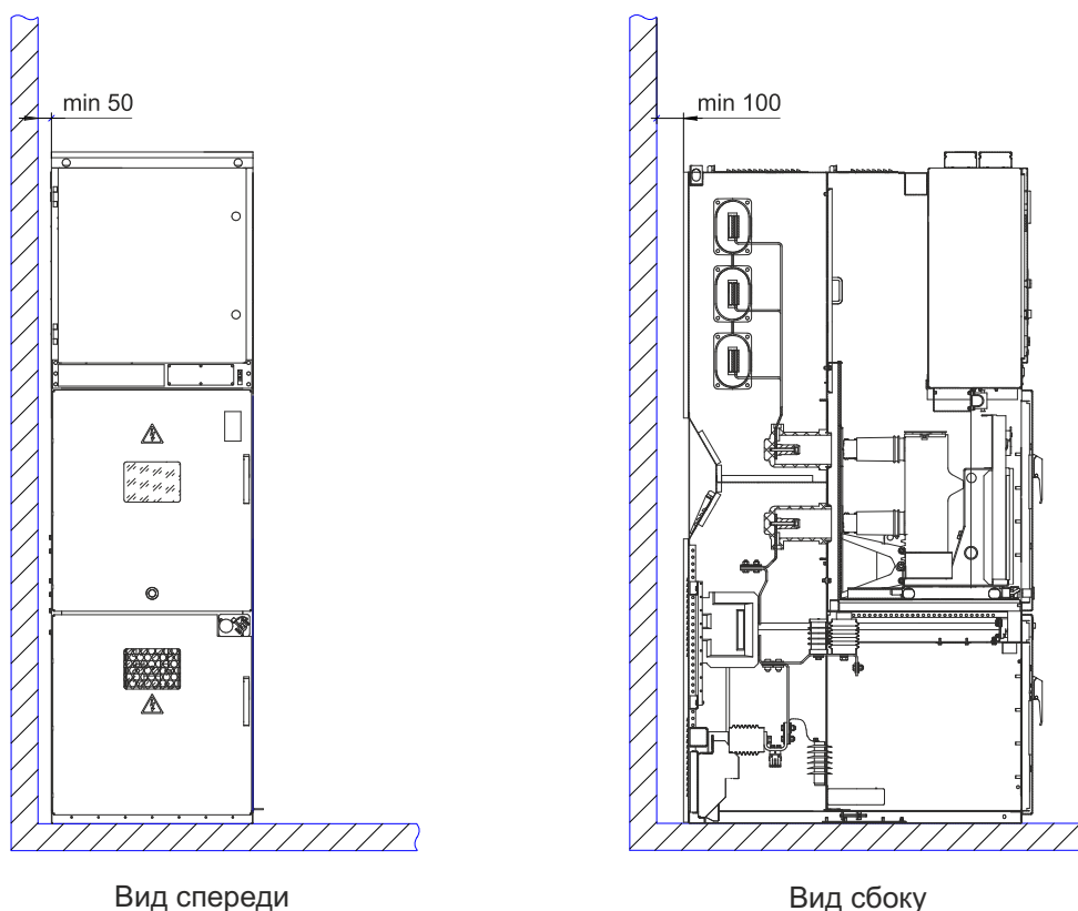
Рис. 6.2 Расположение ячеек в здании
