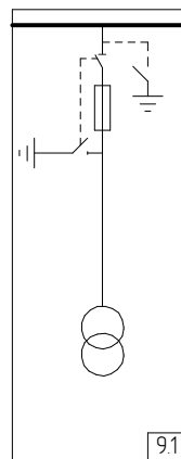
Шкаф с тр-ом собственных нужд (с шинным заземлителем). Подключение на сб-шины.
