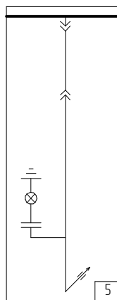
5 Шкаф с разъединителем. Ввод/вывод шинами сзади.
