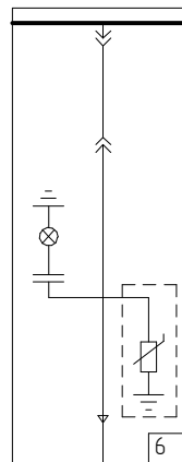
Шкаф с разъединителем. Ввод/вывод кабелем вниз.
