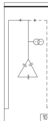
Шкаф с конденсаторной батареей. Подключение кабелем сбоку.
