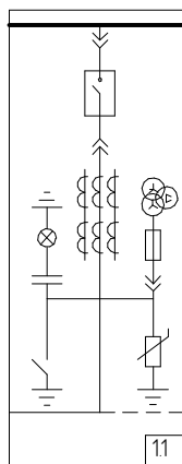
1.1 Шкаф с силовым выключателем и измерительным тр-ом. Ввод/вывод шинами сбоку.
