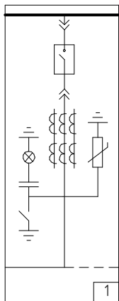
Шкаф с силовым выключателем. Ввод/вывод шинами сбоку.
