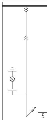
Шкаф с разъединителем. Ввод/вывод шинами сзади.
