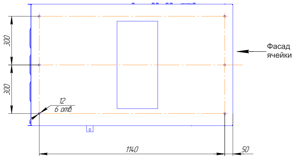
Рис. 6.1 Крепление к полу
