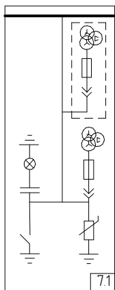
Шкаф с шинным заземлителем, измерительным тр-ом и опломбированным отсеком учета.
