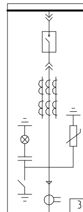
Шкаф с силовым выключателем. Ввод/вывод кабелем снизу.
