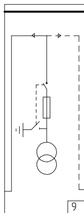
Шкаф с тр-ом собственных нужд. Подключение кабелем сбоку.
